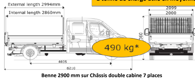
Benne 2900 mm sur Châssis double cabine 7 places
