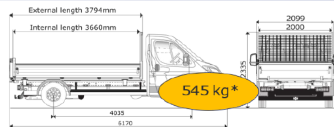
Benne 3700 mm sur Châssis cabine L3 / L
