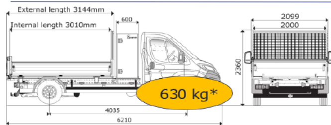
Benne 3050 mm avec coffre sur Châssis cabine L3 / L Option coffre : SP28 / A2R
