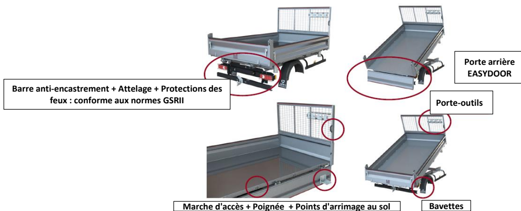
Benne 3050 mm avec coffre sur Châssis cabine L3 / L Option coffre : SP28 / A2R
