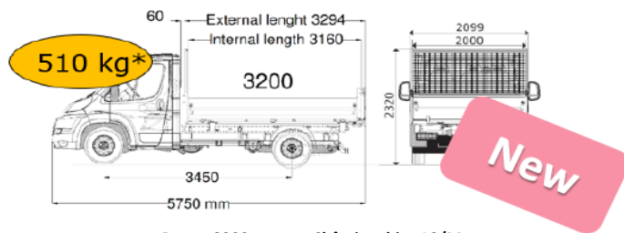
Benne 3200 mm sur Châssis cabine L2/M
